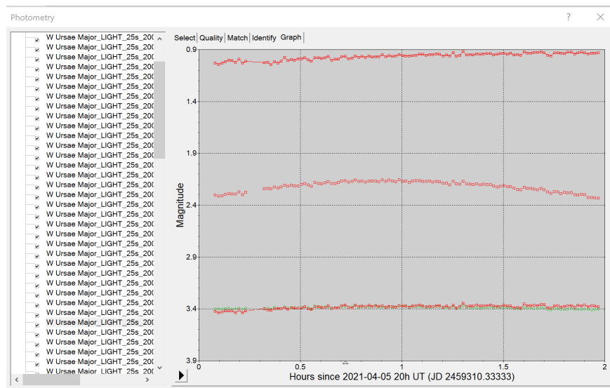
Abb. 1: Die Kurve in der Mitte zeigt die Veränderung der Helligkeit des Sternes W Ursae Majoris über zwei Stunden. Insgesamt wurden mehr als 170 Einzelbilder ausgewertet. Die Punkte ober- und unterhalb sind die Werte von Kontrollsternen.
