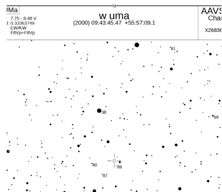
Abb. 3: Eine Karte mit der Helligkeit von Vergleichssternen.
