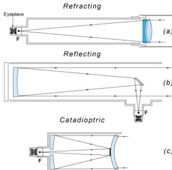
Abb. 1: Verschiedene Bauarten von Teleskopen: a) Linsenteleskop, b) Spiegelteleskop nach Newton, c) Spiegellinsenteleskop.
