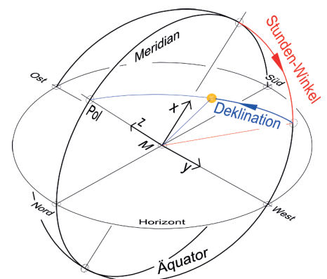
Koordinatensystem mit Kugelkoordinaten (Quelle: Wikipedia)
